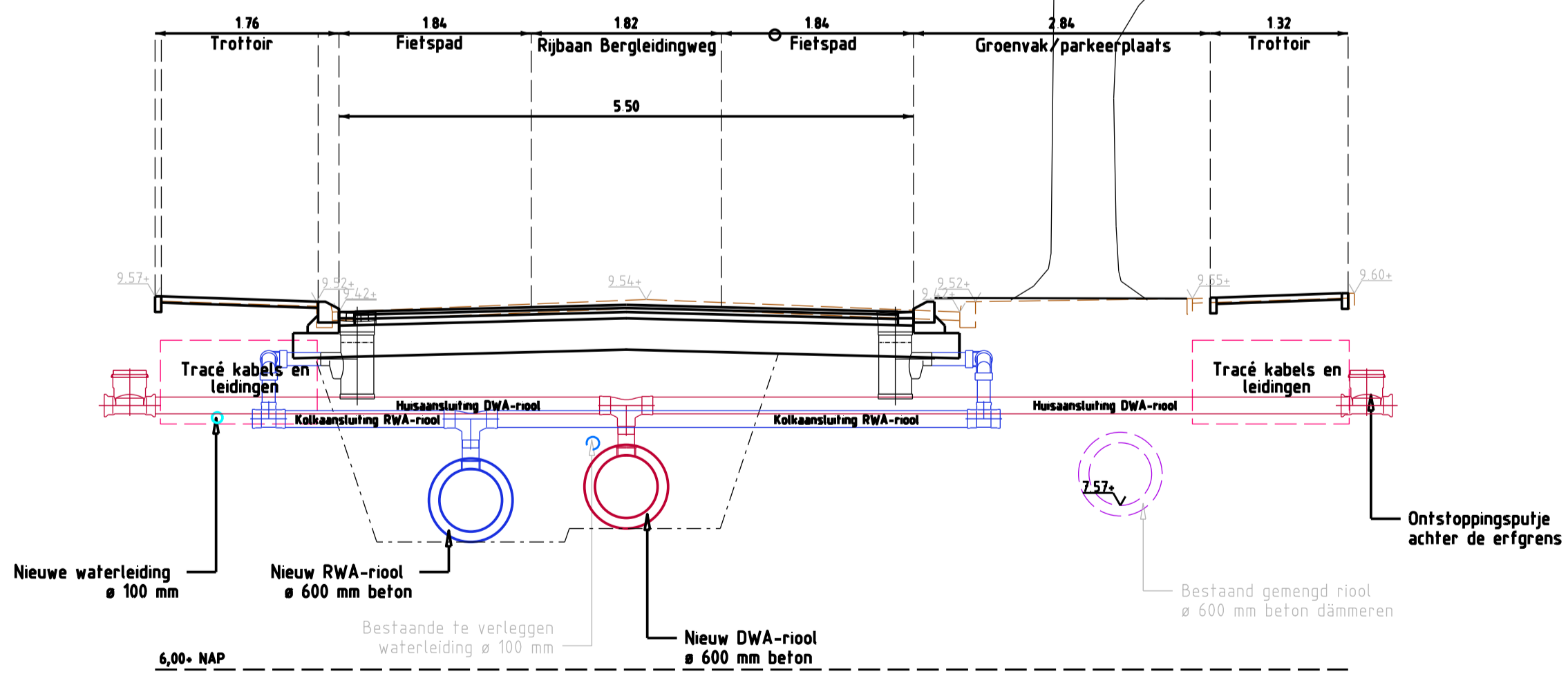
PRINCIPE PROFIEL BERGLEIDINGWEG SCHAAL 1:50
